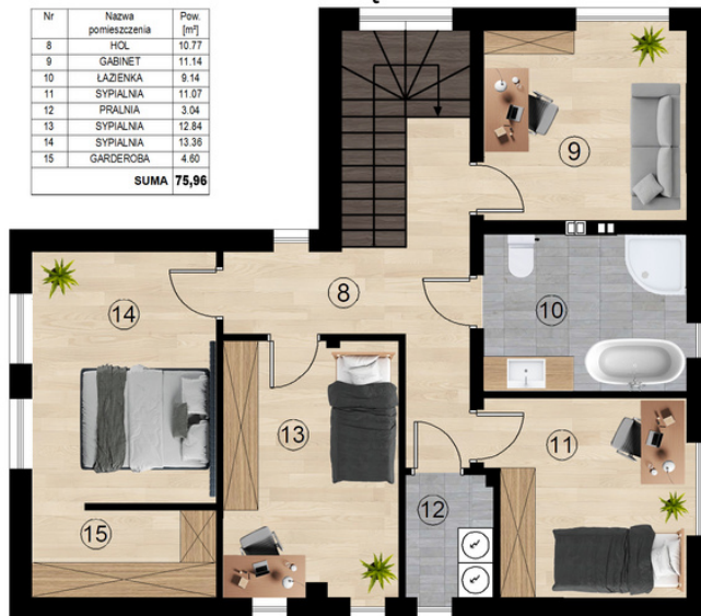
PIĘTRO
